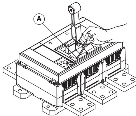
Figure 19 : Bouton pousser-pour-déclencher
